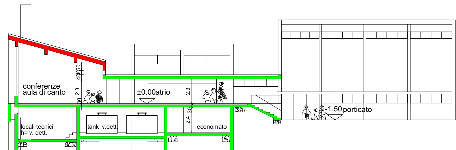
sezione b-b
